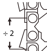
Paso de la cadena 0.325" (8.25 mm)
